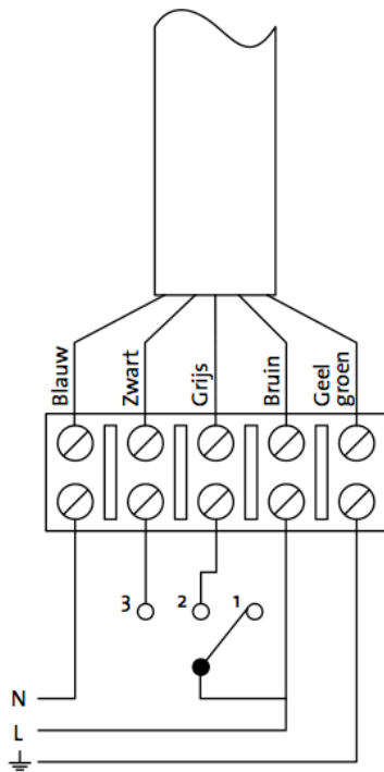
Pijpdakventilator type CVD
