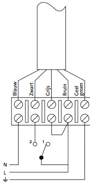
Pijpdakventilator type CVD
